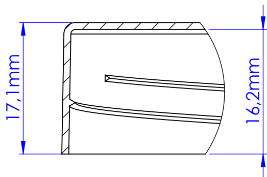
DETALHE B ESCALA 2 : 1
