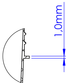
DETALHE B ESCALA 1 : 1
