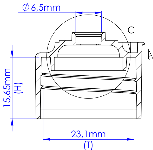
DETALHE B ESCALA 2 : 1
